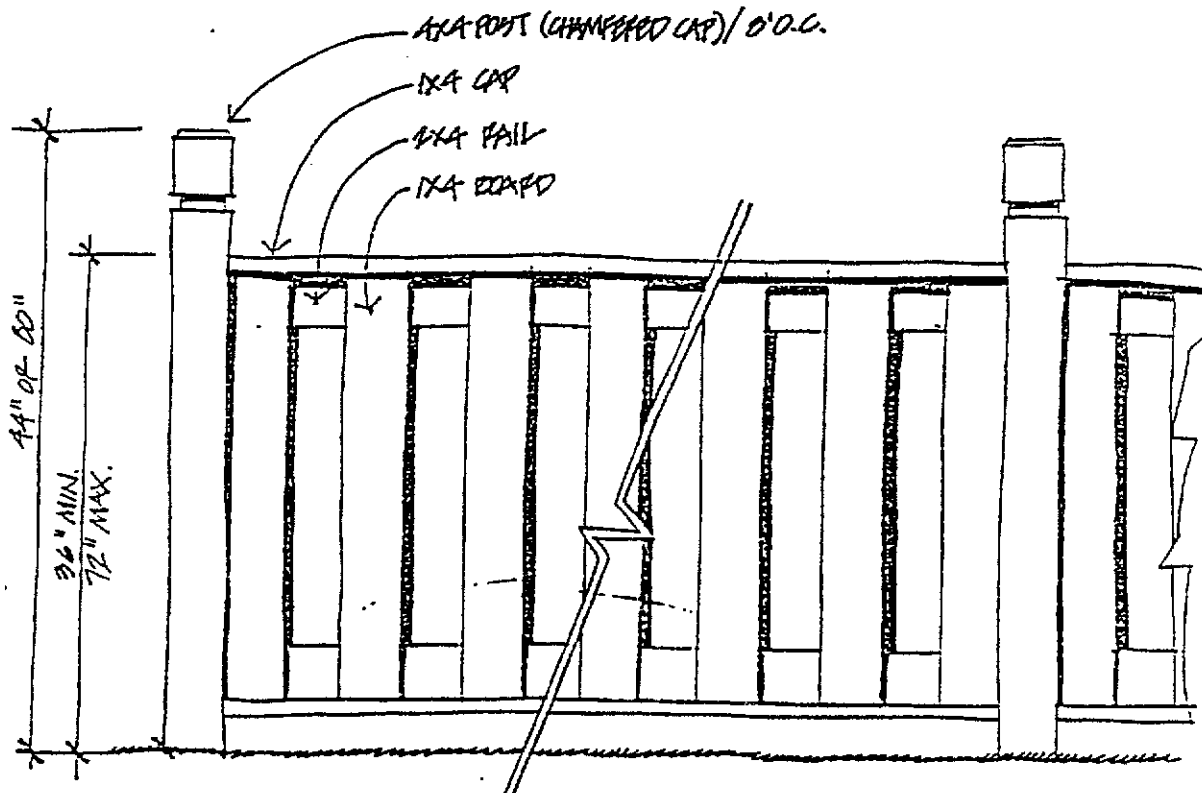
ELEVATION
